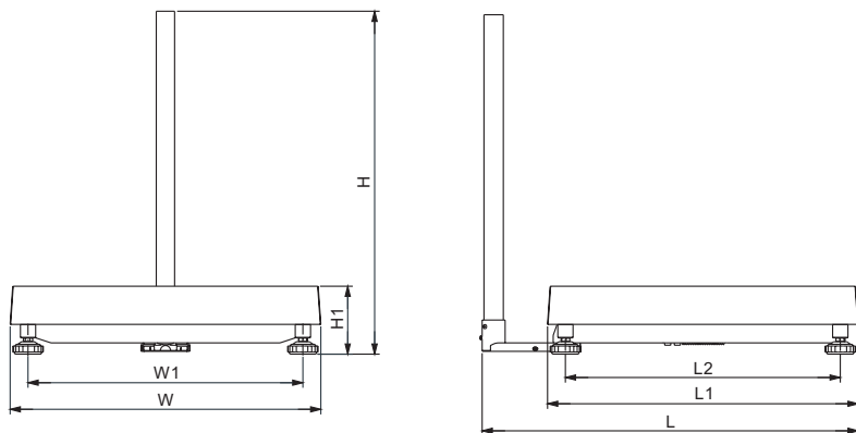
尺 寸(mm)
