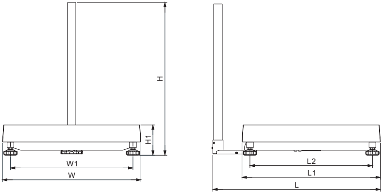
尺 寸(mm)
