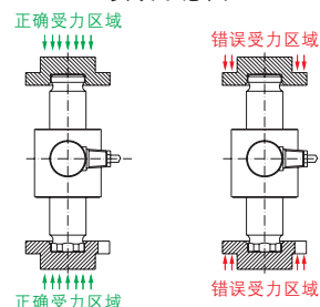
安装示意图:
