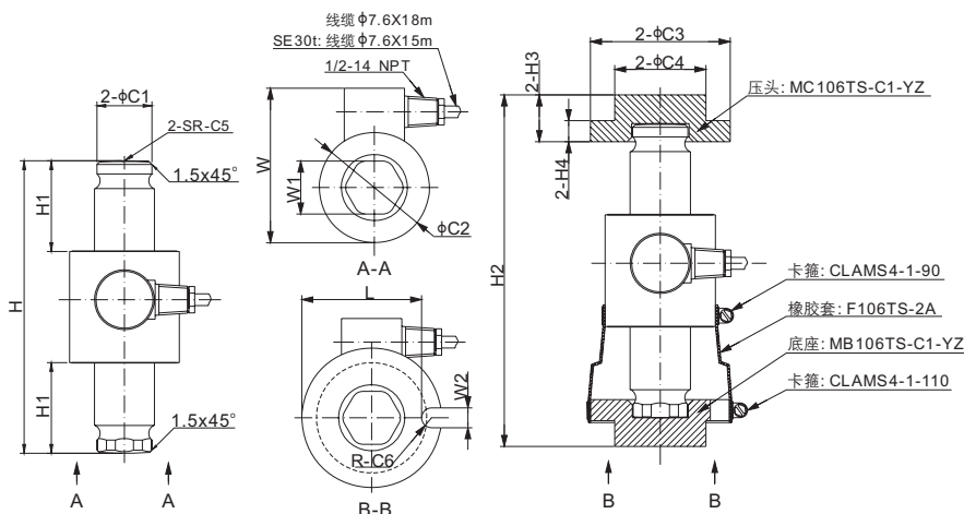
安装示意图:
