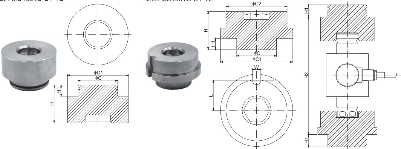
尺 寸
