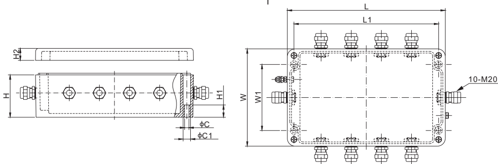
尺寸
