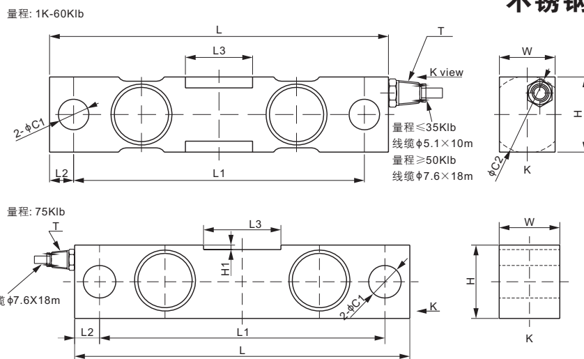
尺寸
